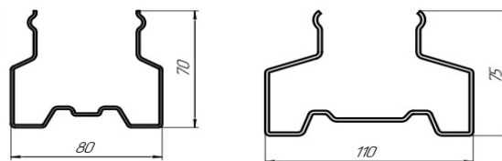
Сечение вертикальных стоек
