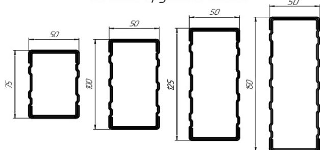
Сечение грузовых балок
